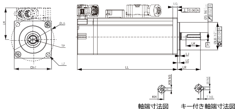
軸端寸法図
